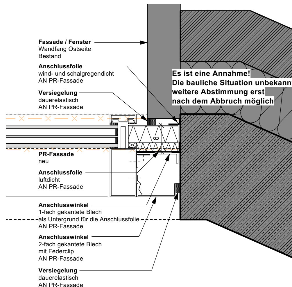
Detail 316-2 Horizontalschnitt PR-Fassade PR 3-1 Erdgeschoss (Ostseite)
