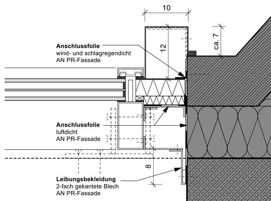
Detail 316-3 Horizontalschnitt PR-Fassade PR 3-2 und PR 4-2 Obergeschoss
