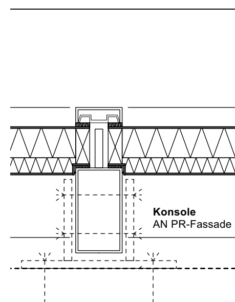
Detail 316-2 Horizontalschnitt PR-Fassade PR 3-1 Erdgeschoss (Ostseite)
